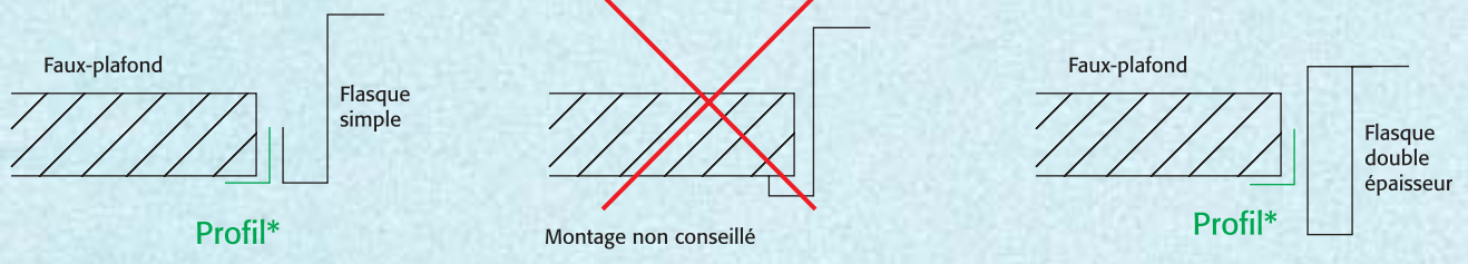
Montage encastré
